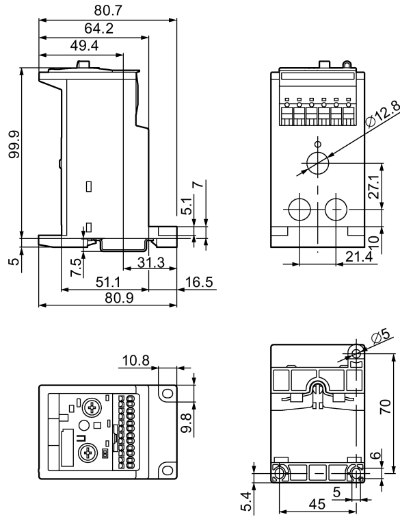
Figure C-26 3RB3.3.-.X.
